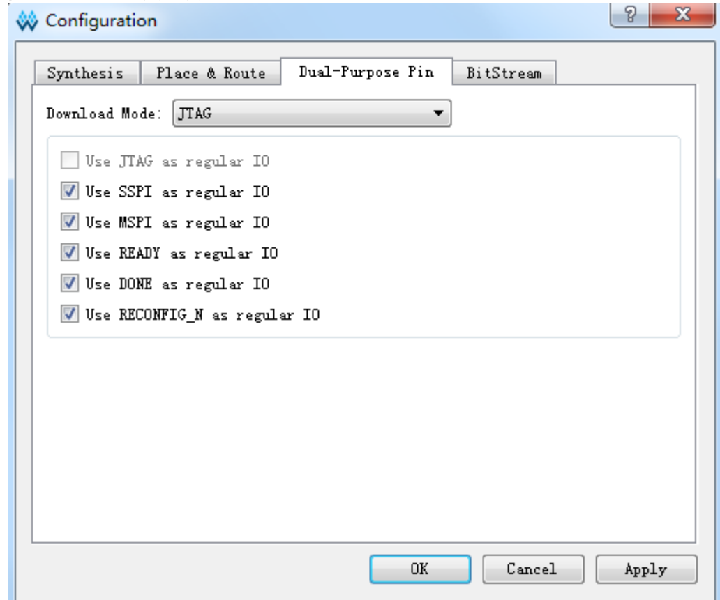
图 3-1 配置管脚复用设置
