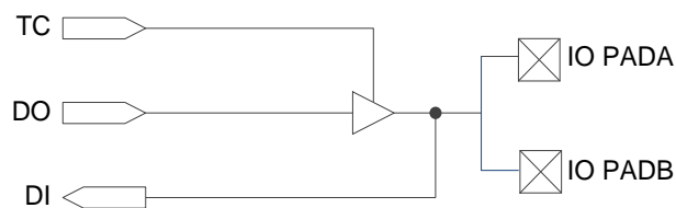
图 7-2 LVDS 输入输出逻辑结构示意图
