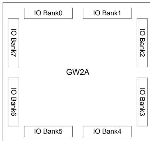
图 4-3 GW2A 系列 FPGA 产品分区分布示意图
