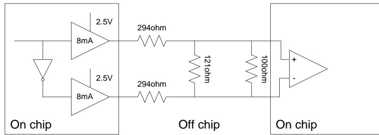
图 8-3 RSDS 匹配网络
