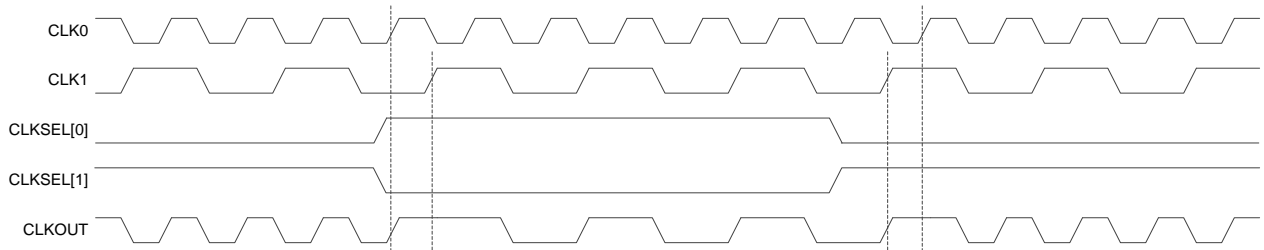
图 3-5 DCS Rising Edge 模式下的时序示意图
