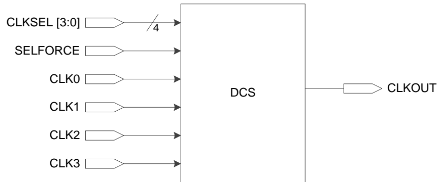
图 3-4 DCS 接口示意图
