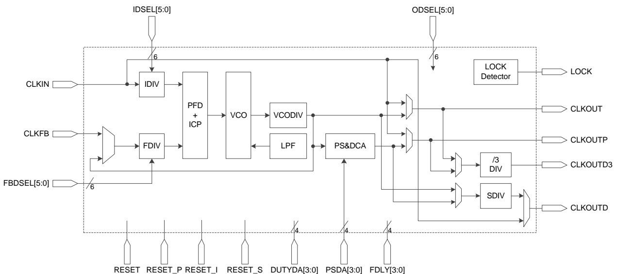
图 7-1 PLL 示意图
