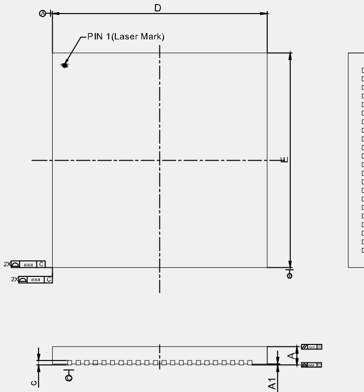
图 4-1 封装尺寸 QN88
