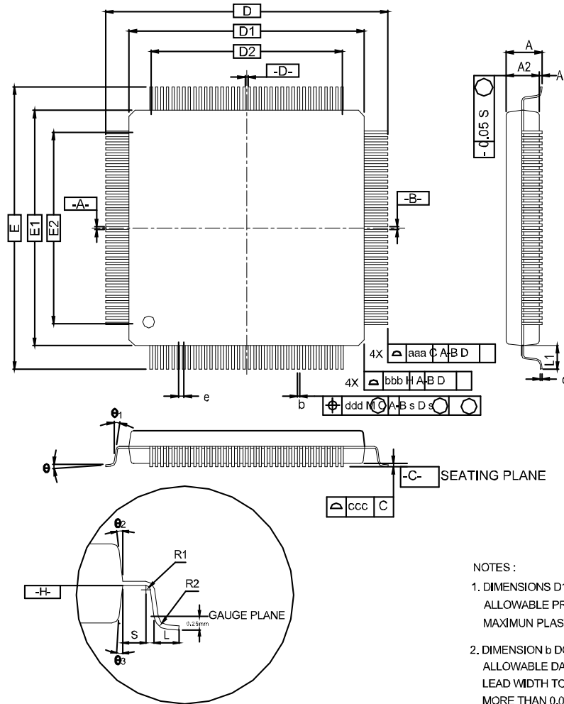
图 4-2 封装尺寸 LQ144
