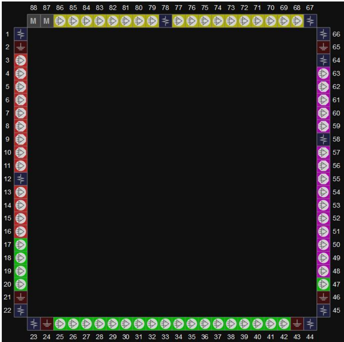
图 3-2 GW1NR-9 器件 QN88 封装管脚分布示意图（顶视图）
