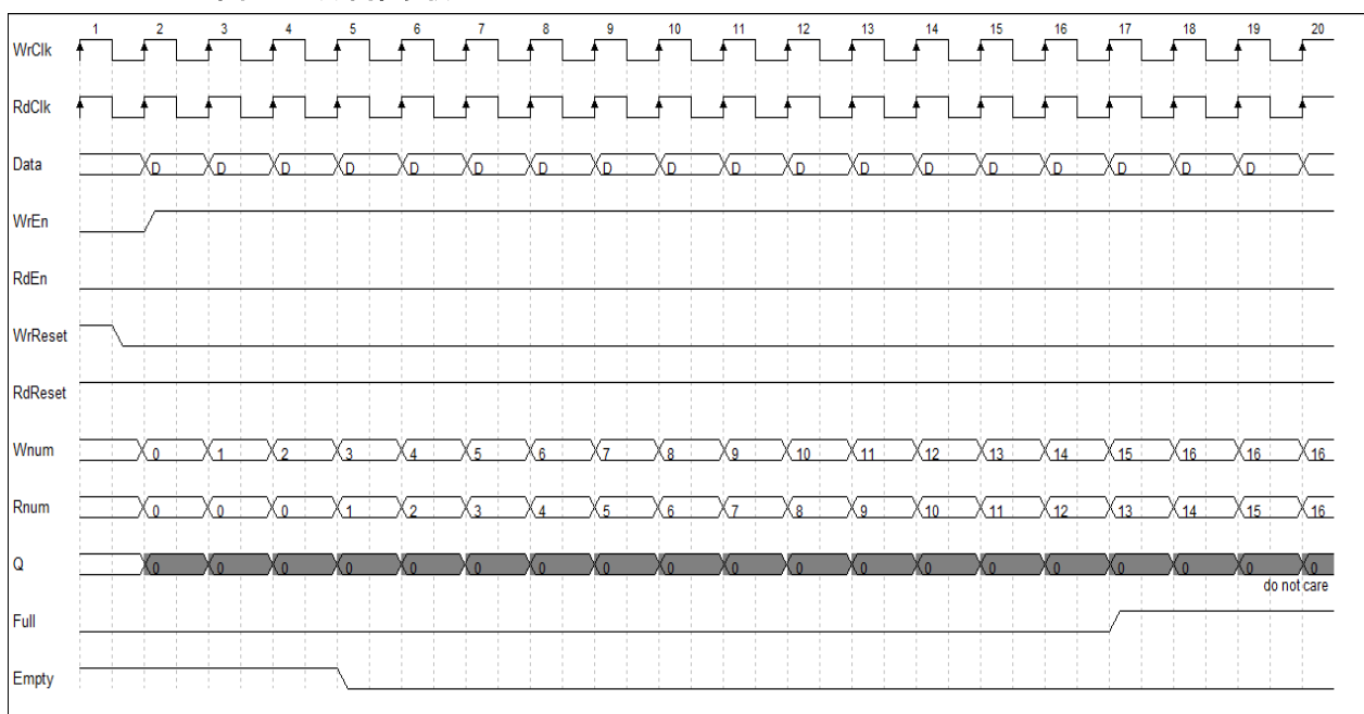
图 4-1 写操作示例
