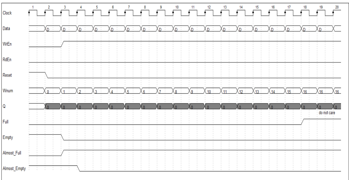
图 4-7 FIFO 满标志和将满标志时序图
