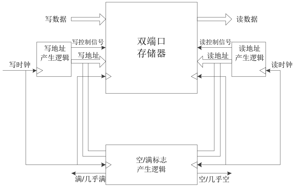
图 2-1 异步 FIFO 结构示意图
