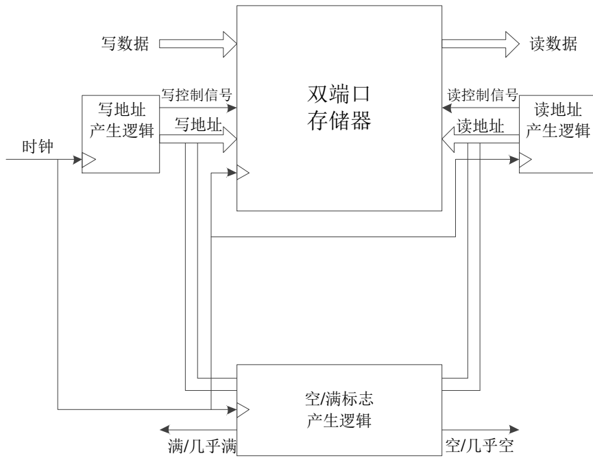
图 2-2 FIFO_SC 结构示意图
